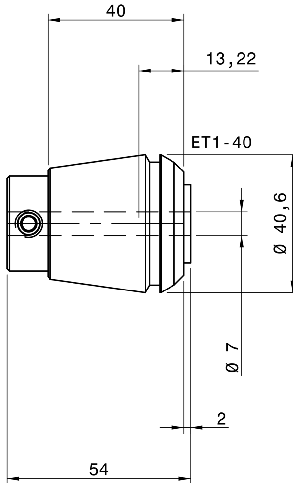
REGO-FIX 1540.07000
