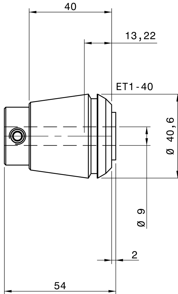
REGO-FIX 1540.09000
