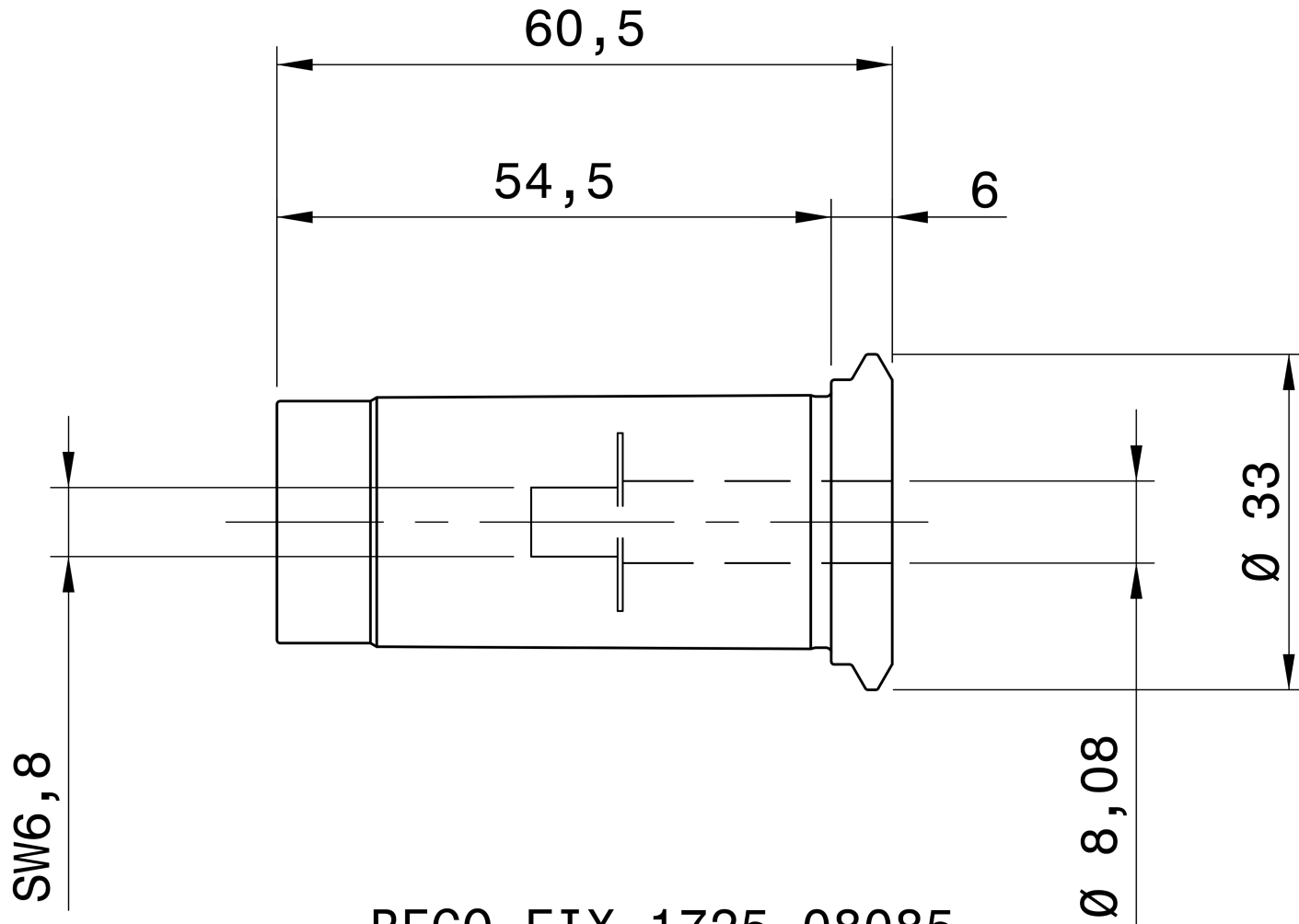
REGO-FIX 1725.08085
