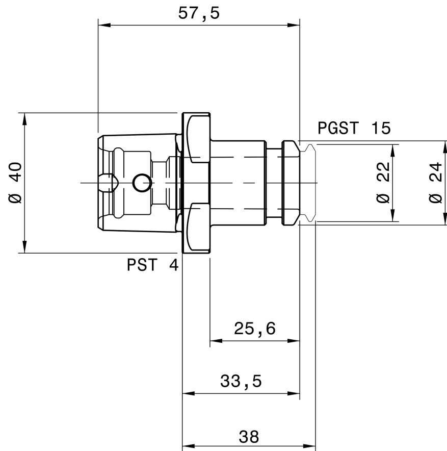
REGO-FIX 2804.71500
