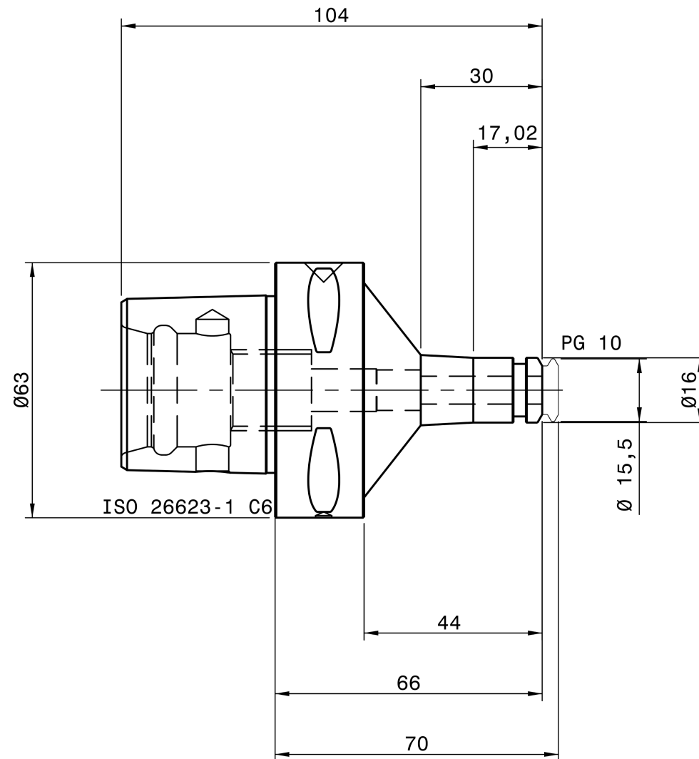
REGO-FIX 2806.71030
