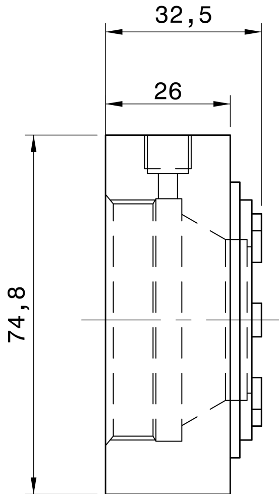
ISO 15488 ER 40 REGO-FIX 3740.19000
