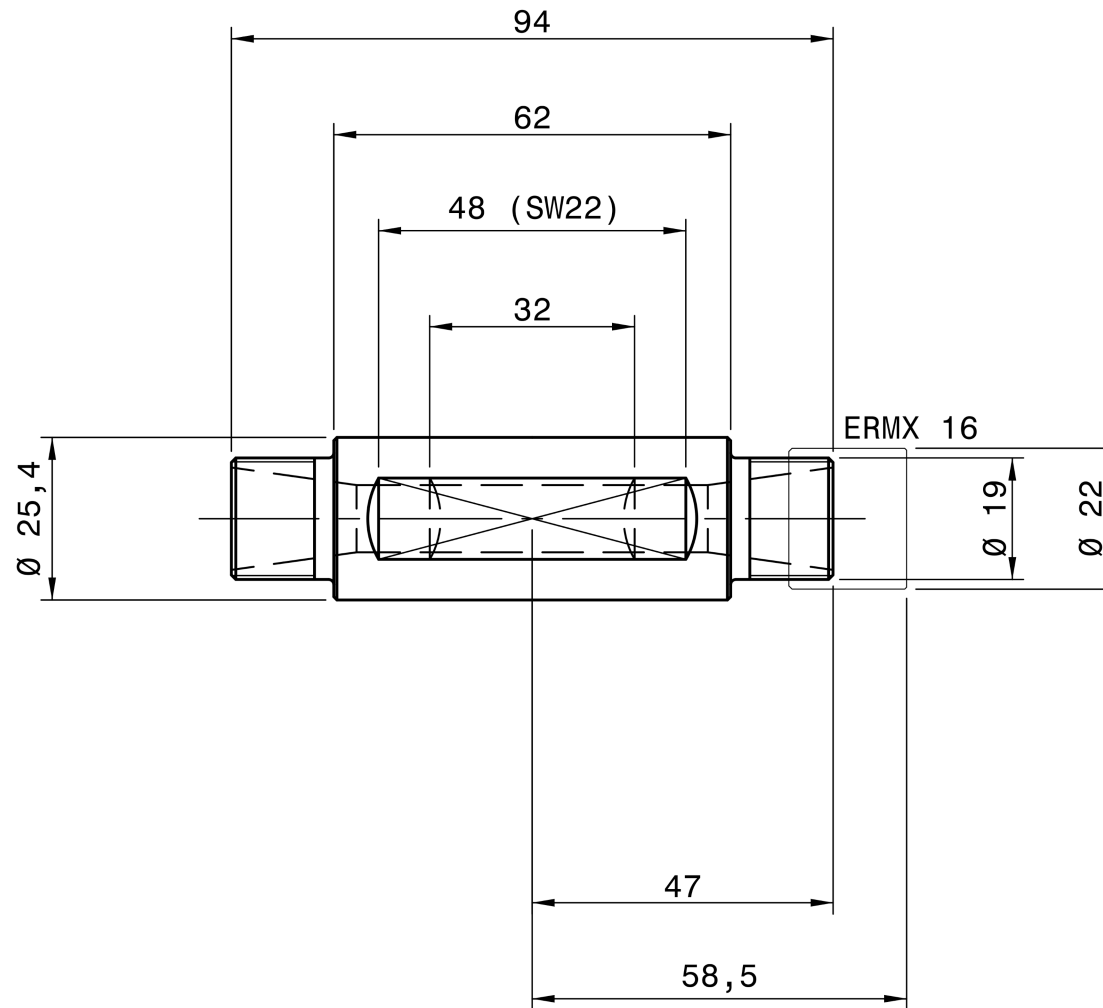
REGO-FIX 4625.21635
