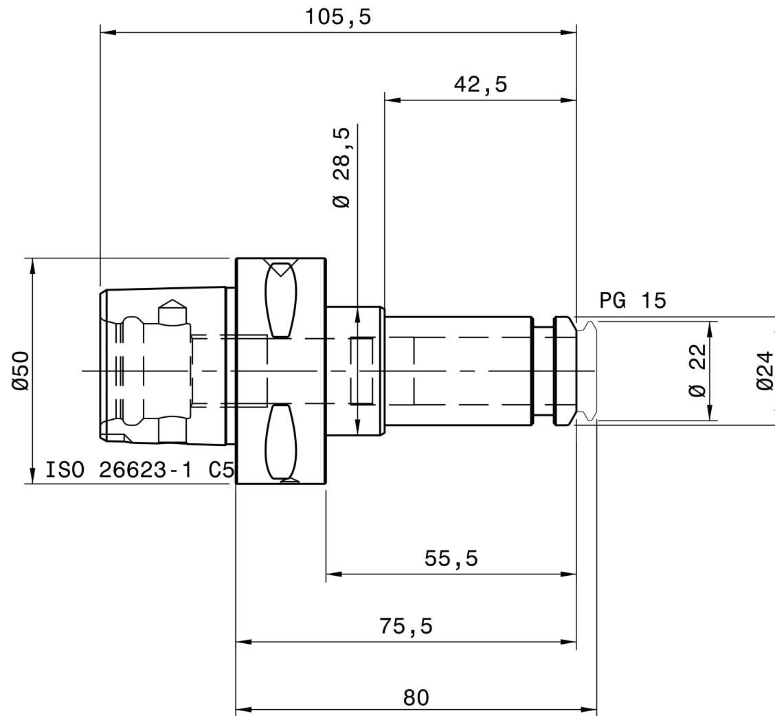
REGO-FIX 4805.71540
