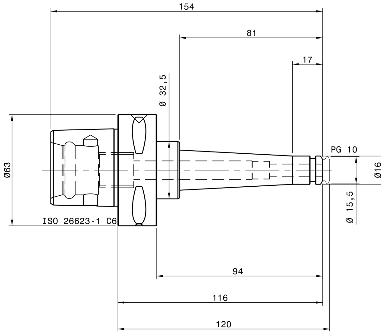
REGO-FIX 4806.71060
