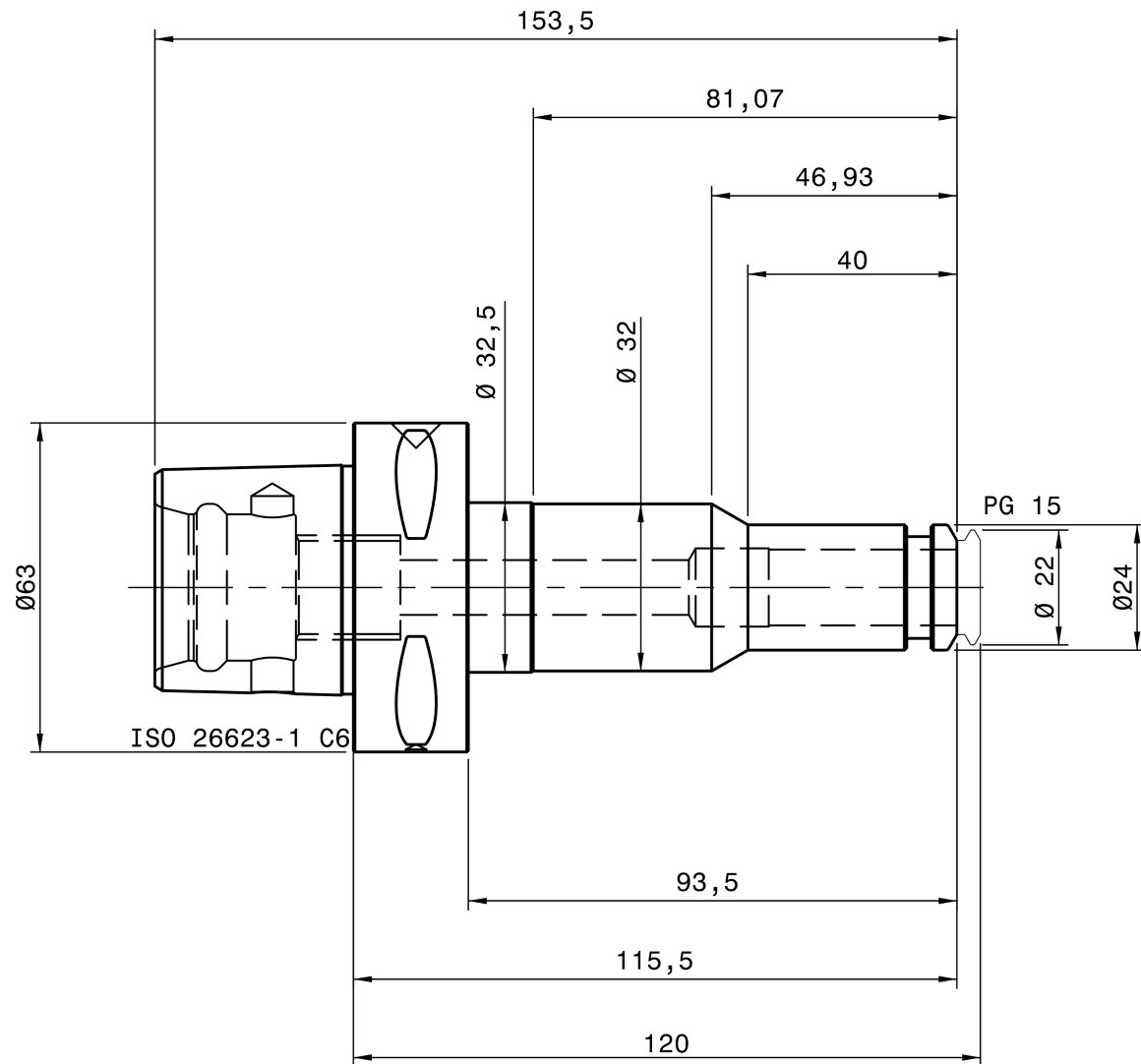
REGO-FIX 4806.71560
