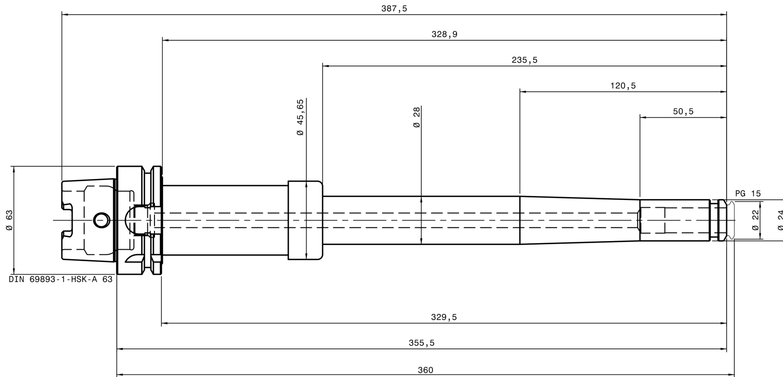
REGO-FIX 8865.73190
